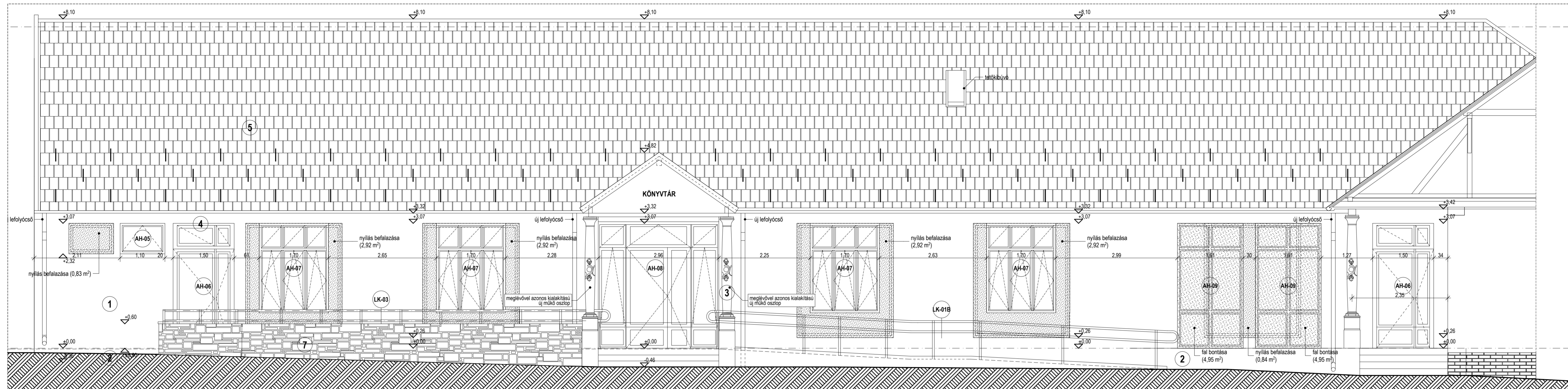
ÉSZAK-KELETI HOMLOKZAT (1) 1:50
