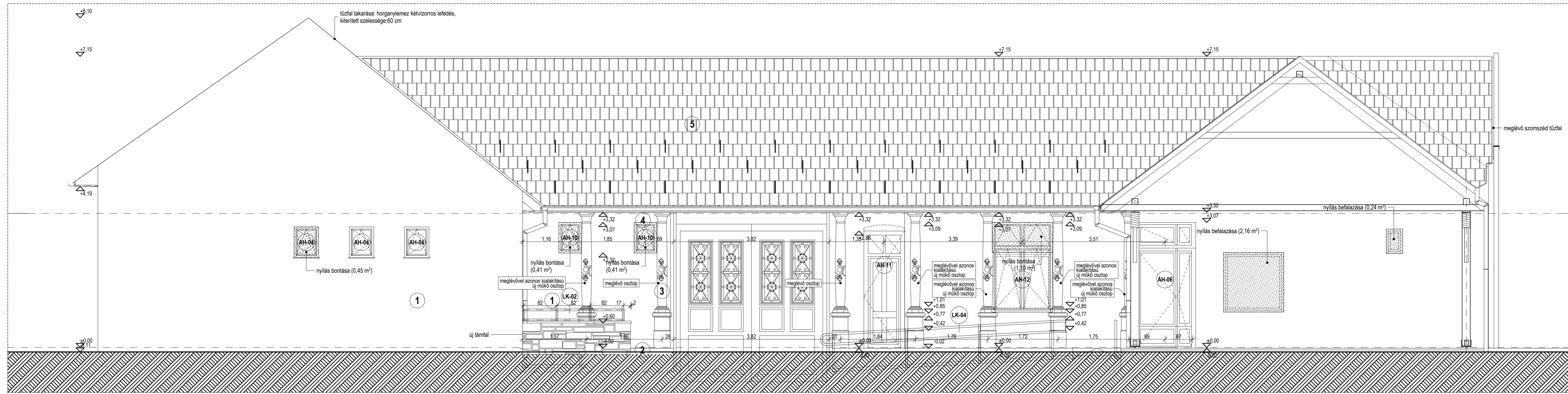
DÉL-KELETI HOMLOKZAT 1:50
